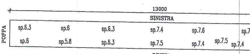
ZATTERINO DI POPPA SINISTRA - FONDO
