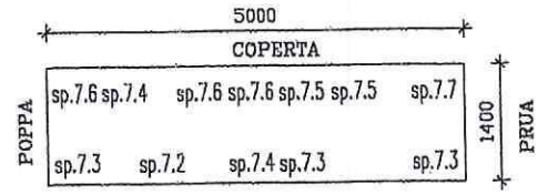
ZATTERINO DI PRORA DRIFFA
