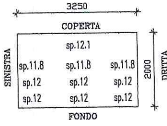
SPECCHIO DI POPPA
