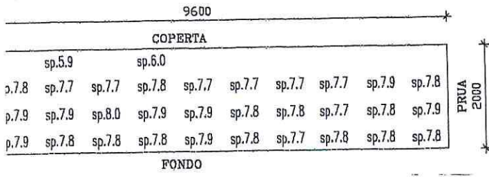
MACCHINE LATO DRIFFO
