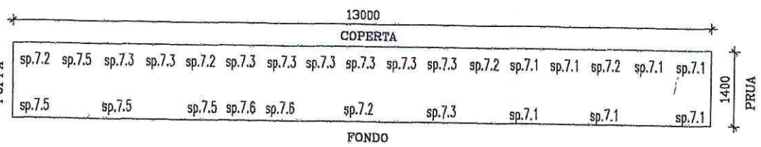
ZATTERINO DI POPPA DRIITA - FIANCATA DESTRA ESTERNA
