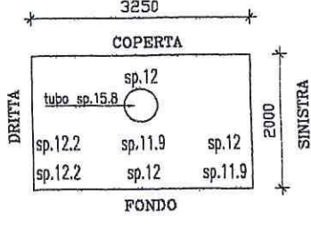
SPECCHIO DI PRORA
