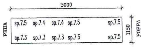
ZATTERINO DI PRORA DRIFFA-FONDO
