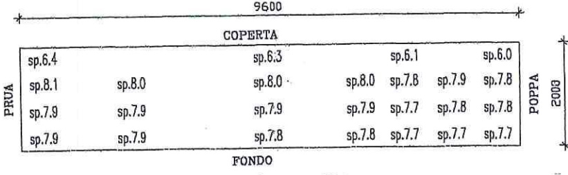
SALA MACCHINE LATO SINISTRO
