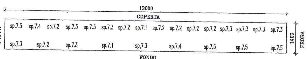
ZATTERINO DI POPPA DRIITA - FIANCATA SINISTRA INTERNA
