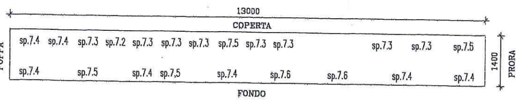
ZATTERINO DI POPPA SINISTRA - FIANCATA DESTRA INTERNA
