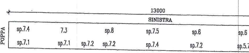
ZATTERINO DI POPPA DRIITA - FONDO
