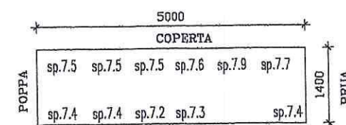
ZATTERINO DI PRORA SINISTRA
